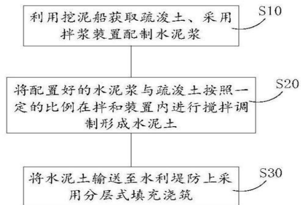
图 2 为实施例的水利堤防的施工方法的流程图。
