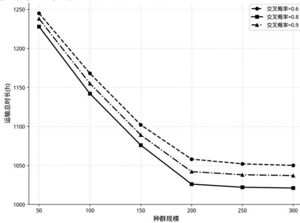
图2 种群规模对运输总时长的影响曲线
