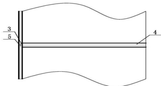
图 2 建于砂卵石地基上的胶结砂砾石坝坝体防渗施工方法中某溢流坝仓面俯视图
