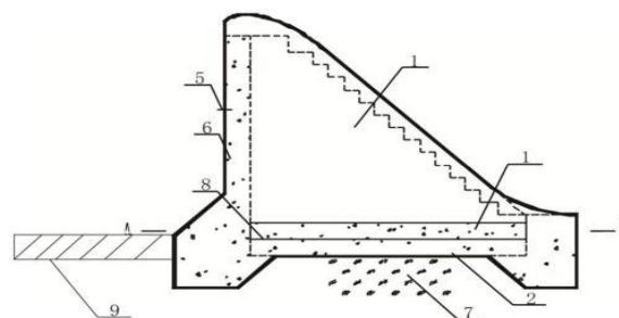
图 1 为建于砂卵石地基上的胶结砂砾石坝坝体防渗施工方法中某溢流坝剖视图
